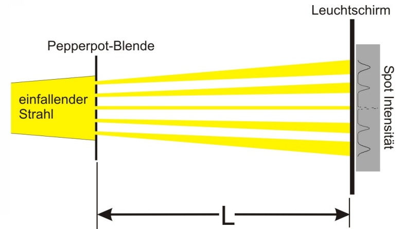
Pepper-pot Emittanzmeßanlage
